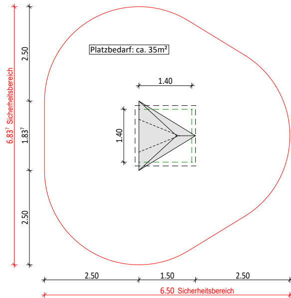
Draufsicht
