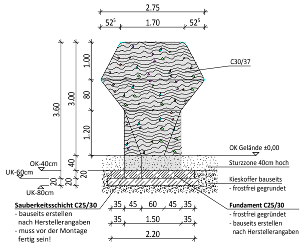
Vorderansicht
