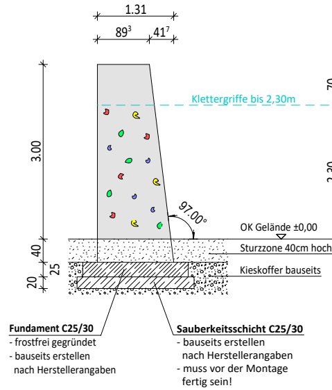
Ansicht B--B
