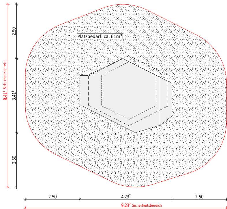
Draufsicht
