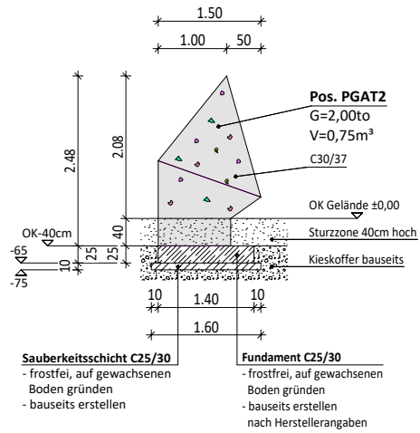
Vorderansicht
