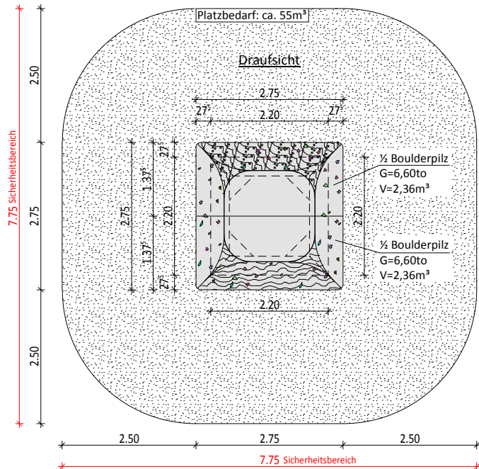
Draufsicht
